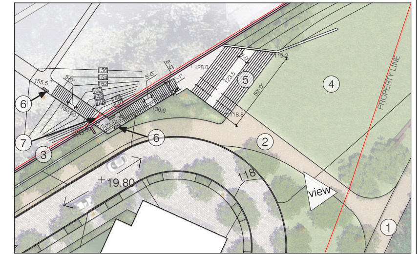
Plan Enlargement
